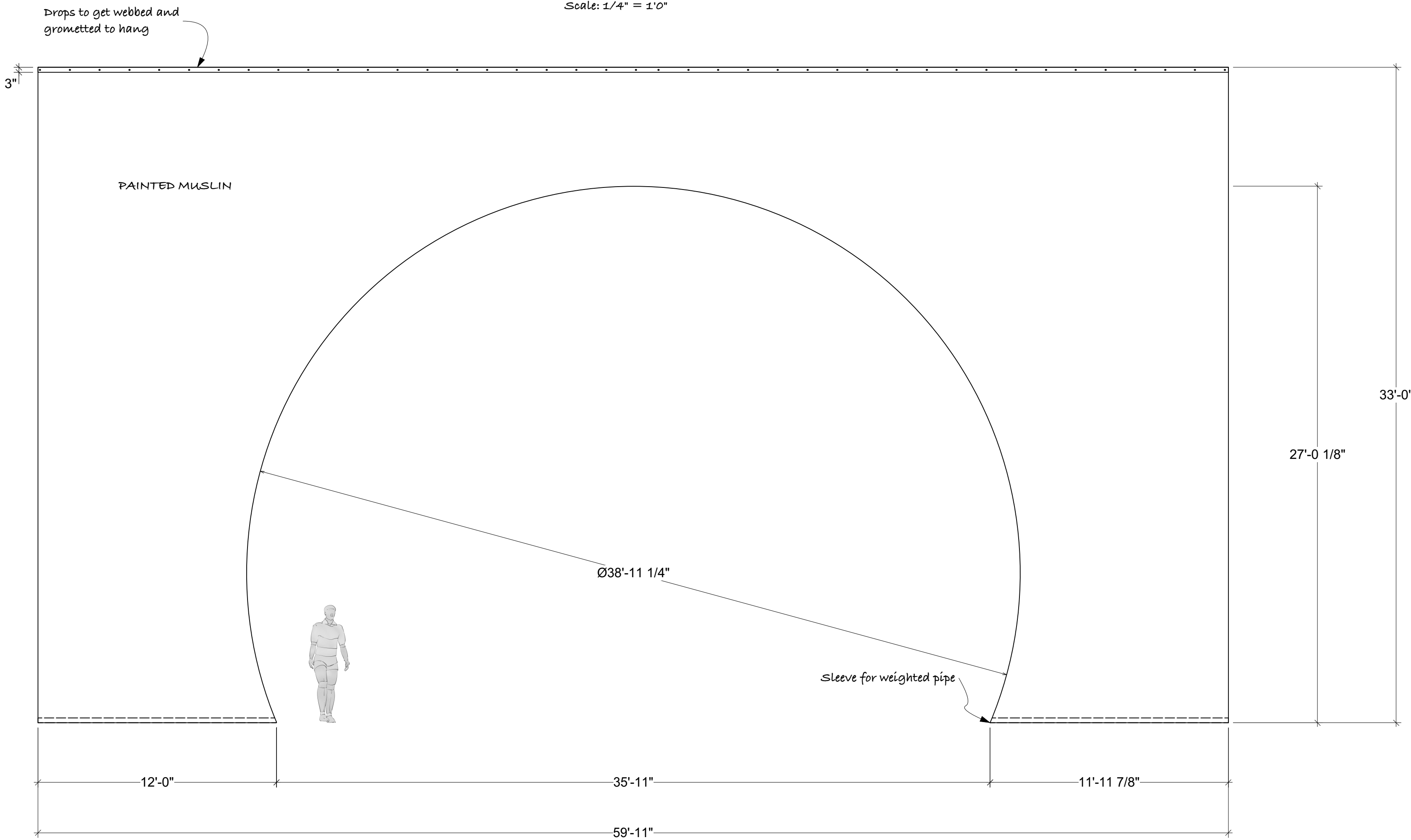
US Portal *** BUILD 3 *** Scale: 1/4" = 1'0"
