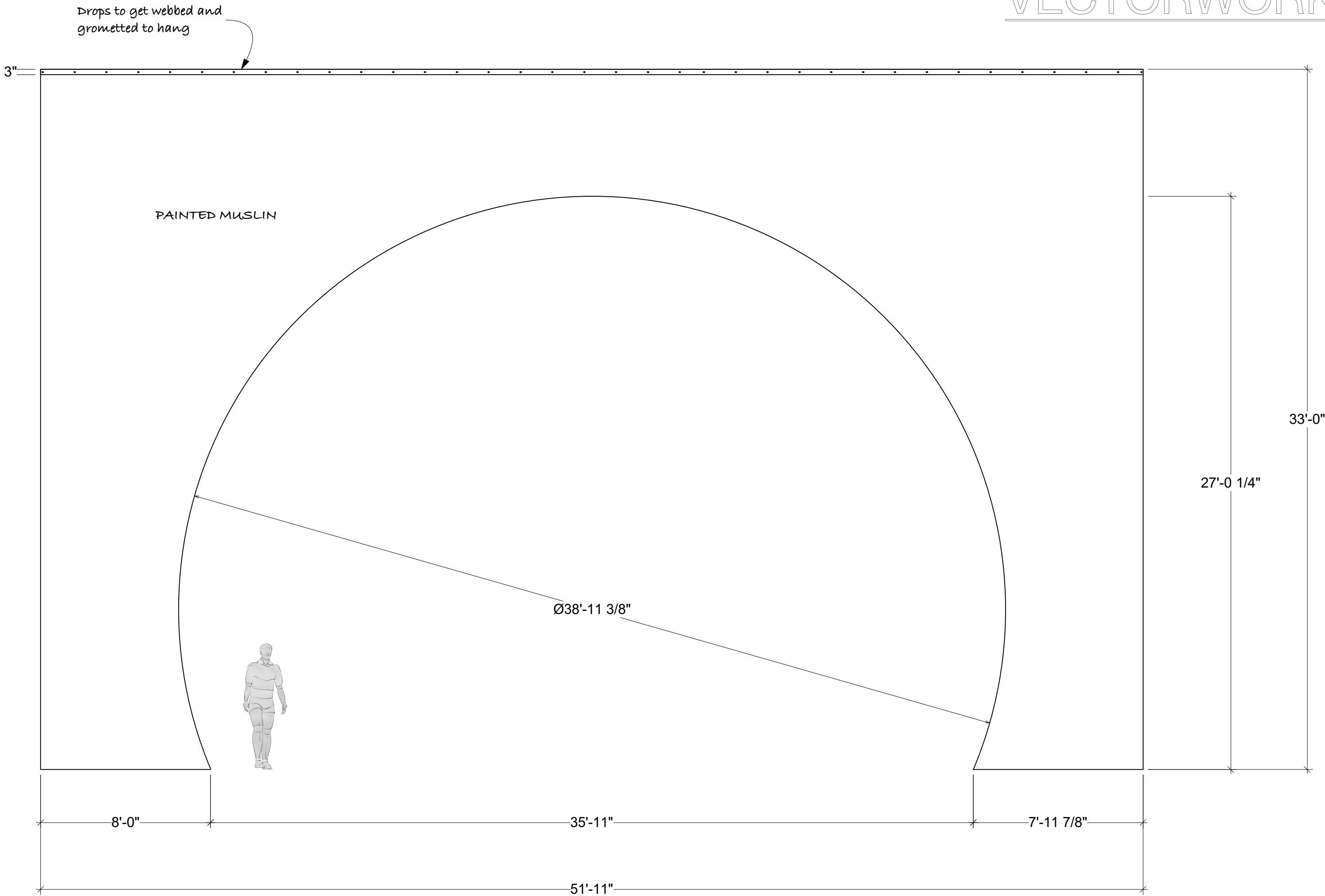
DS Portal Scale: 1/4" = 1'0"
