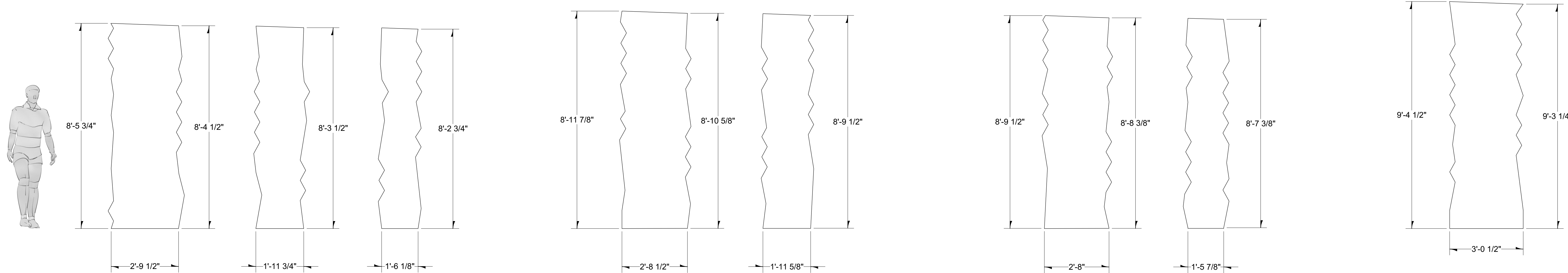
ELEVATION E1
